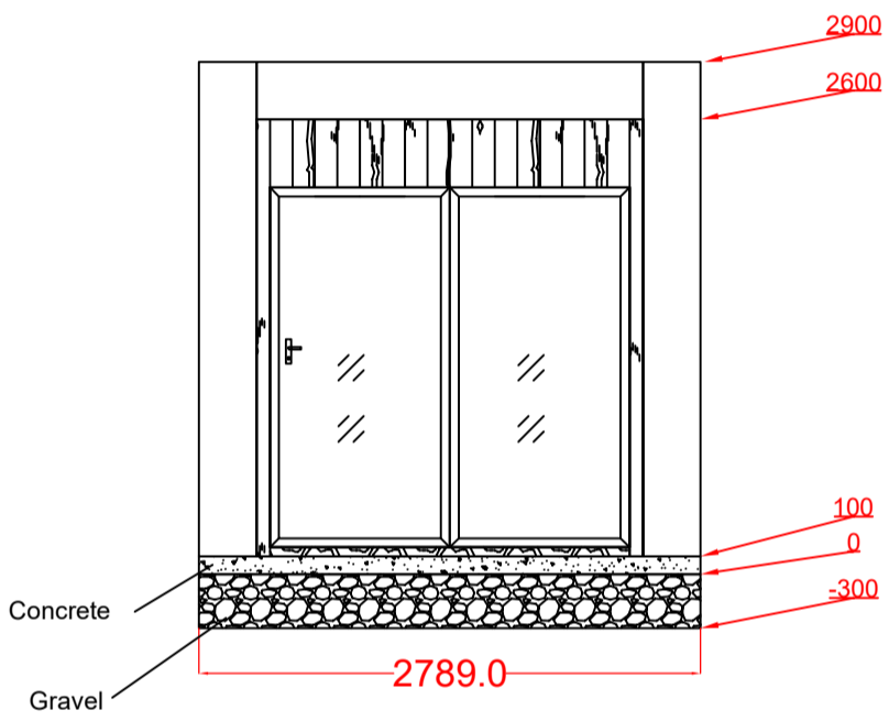
1 Elevation
