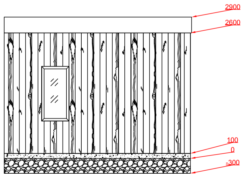
4 Elevation
