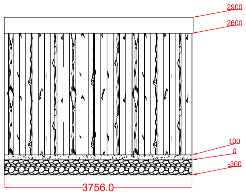
3 Elevation
