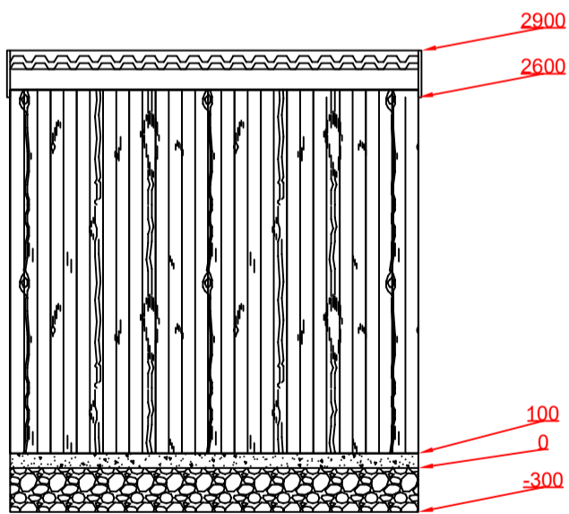
2 Elevation
